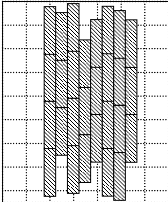
Abb. 3 Verlegung erfolgt kantensetzt zu den Doppelbodenplatten
