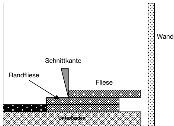
Abb. 2 Zuschnitt der Randfliesen
